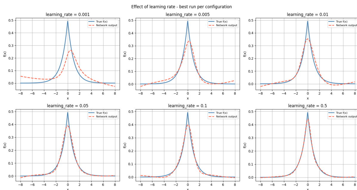
Rys. 4. Wpływ szybkości uczenia się – najlepsze uruchomienie dla danej konfiguracji
